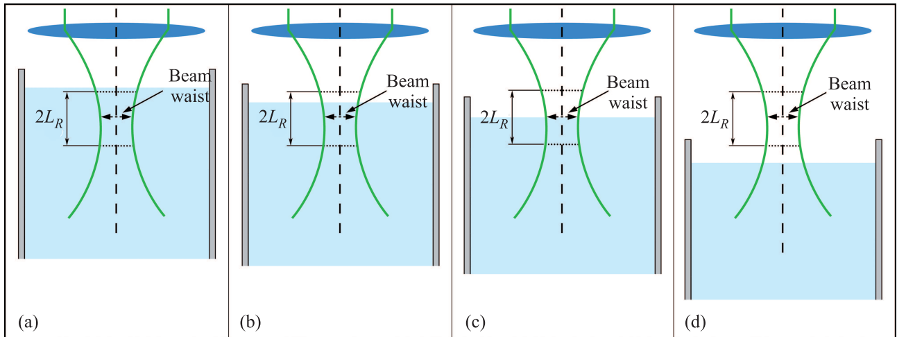
Рис. 3. (Цветной онлайн) Схема положения каустики пучка накачки (удвоенная длина Рэлея 2L_R или конфокальный параметр) относительно поверхности жидкого азота при перемещении дьюара вниз (без учета показателя преломления n = 1.19 жидкого азота [12] и смещения перетяжки [14] в объеме азота)
