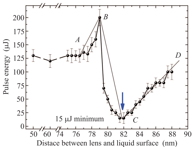
Рис. 2. (Цветной онлайн) Зависимость порога ВКР от расстояния между линзой и поверхностью. Отрезки прямых между точками ABCD соединяют точки начала роста порога, максимального и минимального значения
