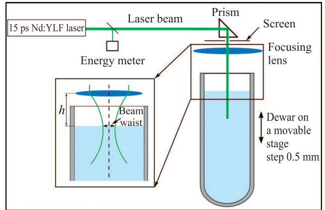
Рис. 1. (Цветной онлайн) Схема эксперимента по изучению аномального снижения порога ВКР 15 пс импульсов (527 нм) в жидком азоте при перемещении каустики пучка через открытую поверхность. На вставке – схема измерения расстояния линза–поверхность
